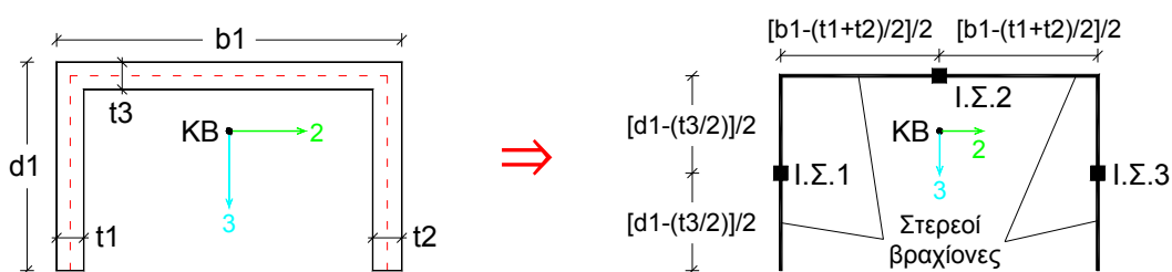
Σχήμα 1. Ισοδύναμο πλαίσιακό προσομοίωμα μονοκυψελικού πυρήνα, το οποίο δημιουργείται αυτόματως από το ΡΑΦ
