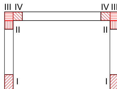
Πίνακας 7. Λόγοι εξάντλησης της ενιαίας διατομής και των σκελών ( q=3.00 )
